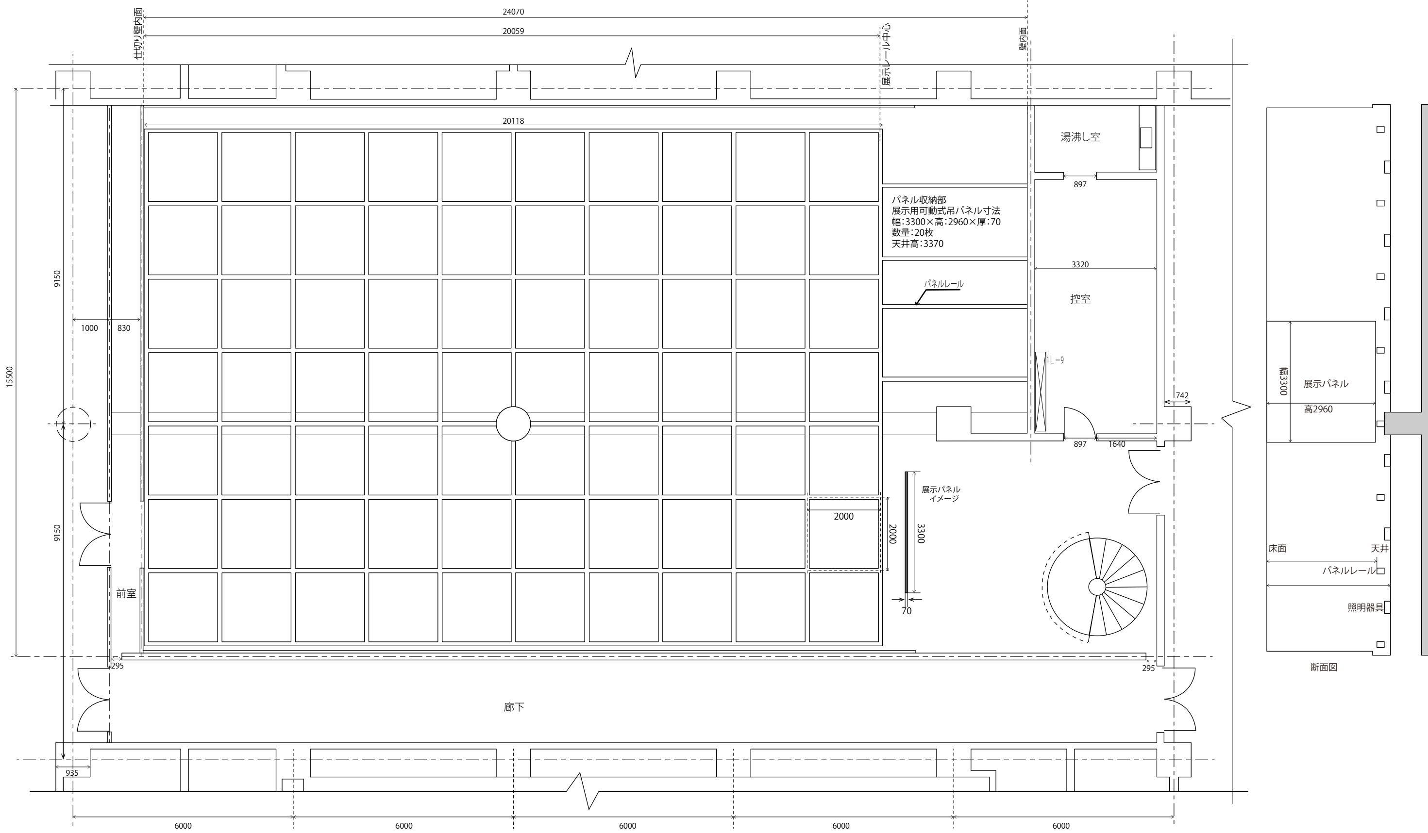
展示室平面図 S=1:100
