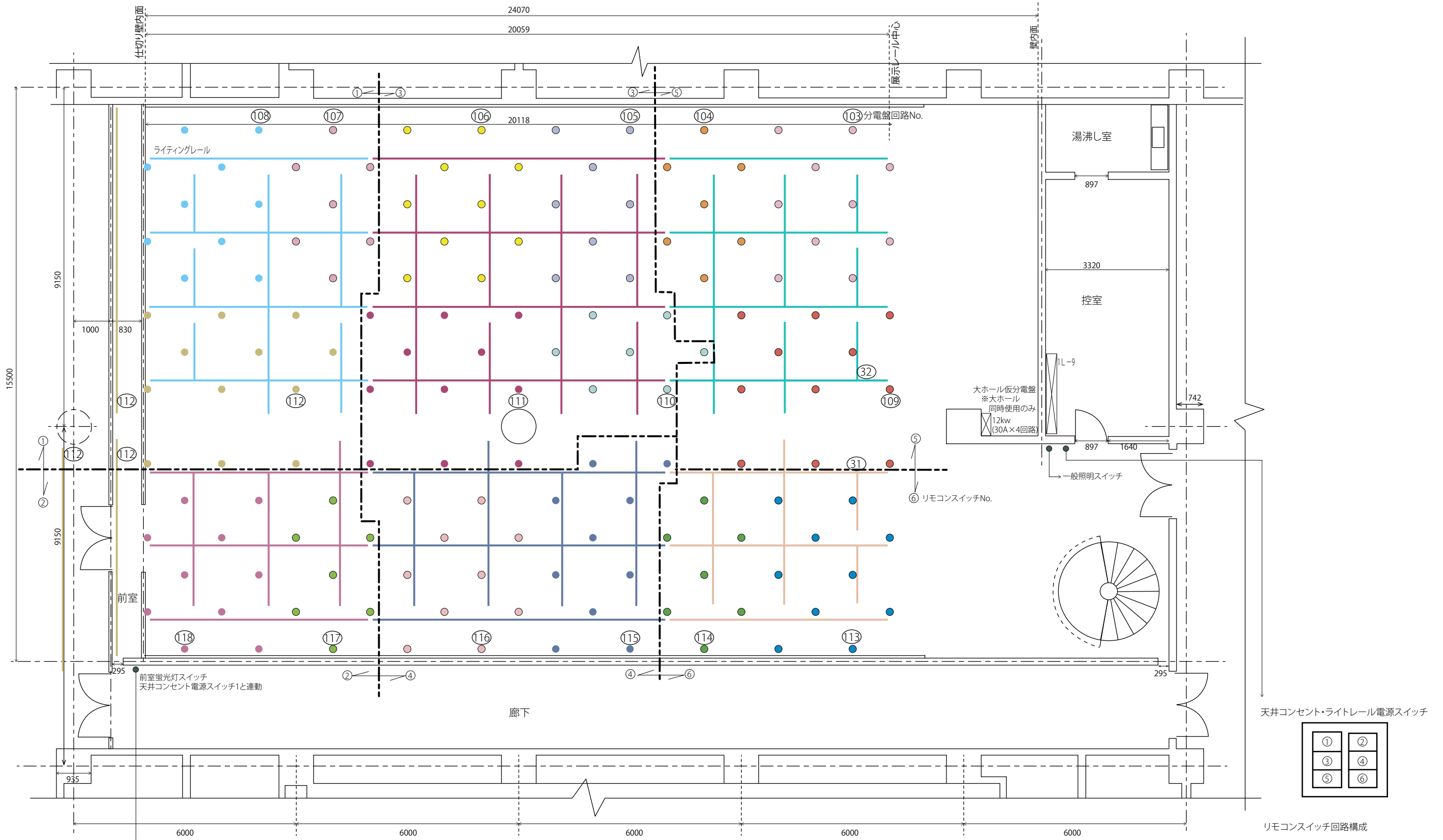
展示室平面図 S=1:100
