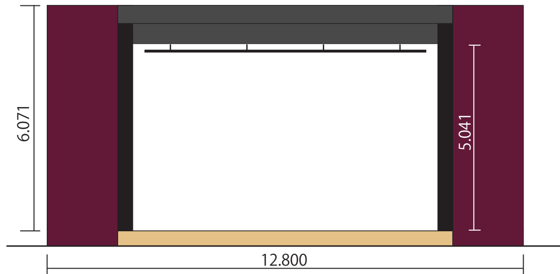
正面図
